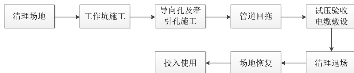
图 2.2-3 电缆拉管敷设施工期工艺流程及产污节点图
