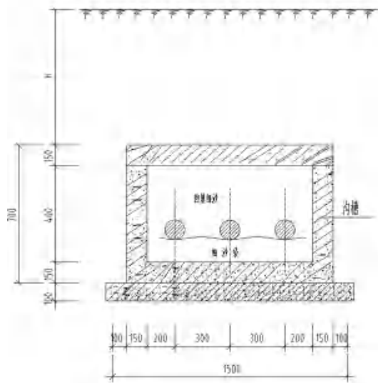
图 2.1-8 电缆沟槽敷设断面图
