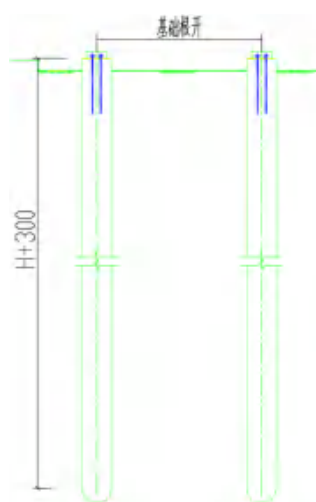
图 2.1-7 基础根开图
